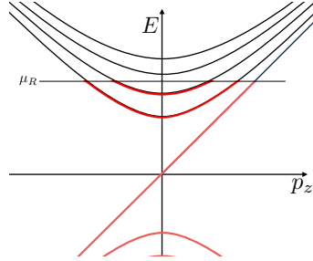
図 7: 右巻き Weyl フェルミオンに磁場をかけ化学ポテンシャルが有限の場合のスペクトル．
