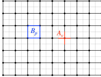
図 10: Toric code に現れる演算子 A_v と B_p .
