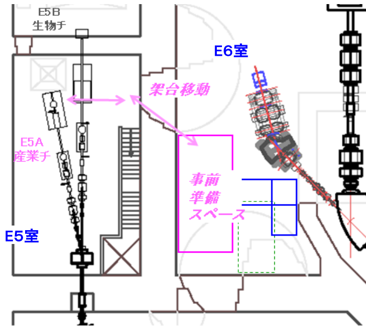
E5~E6 遮蔽扉
