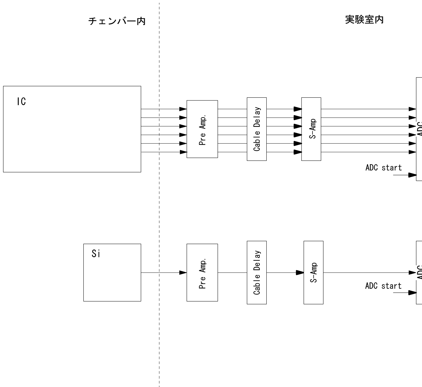
IC and Si 回路図
